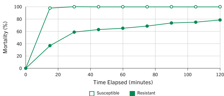
5 Bottle bioassay (15 µg permethrin)
